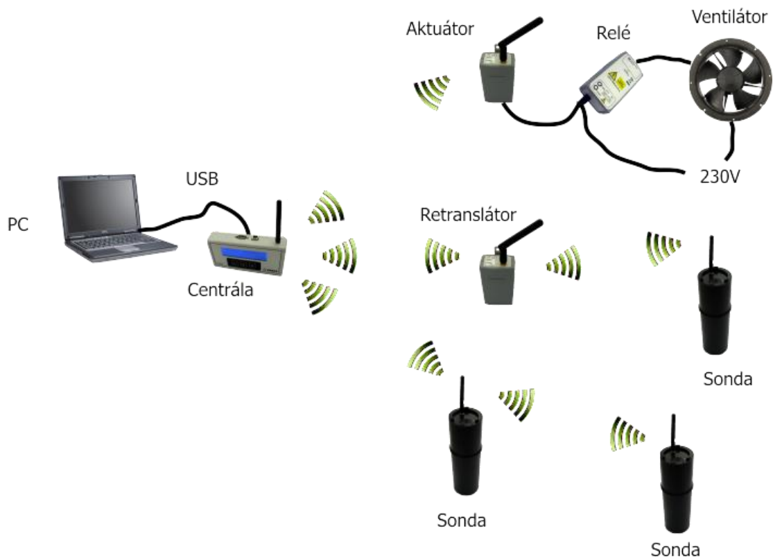
Obrázek 2 - Zapojení centrální jednotky TCR3 v regulačním systému TERA
