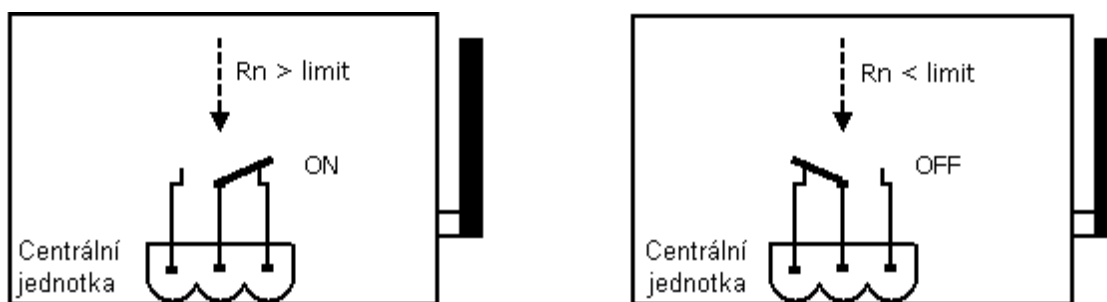
Obrázek 3 - Zapojení výstupních kontaktů konektoru relé
